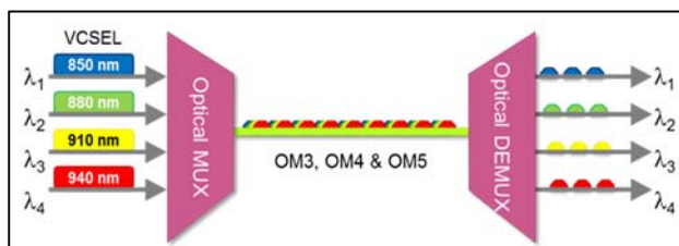
Afb. 4: SWDM-overdracht met vier golflengten in MMF
