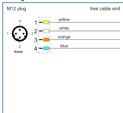
Wiring
